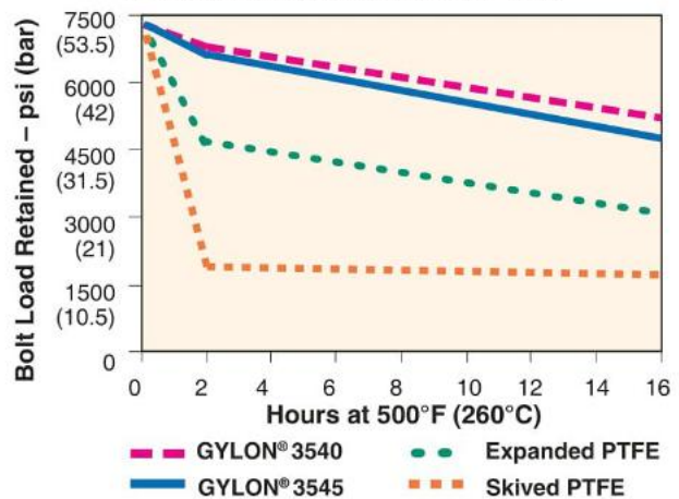
DIN 52913 Gasket Bolt Load vs. Time
